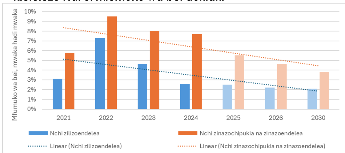
Kielelezo Na. 3: Mfumuko wa bei duniani
